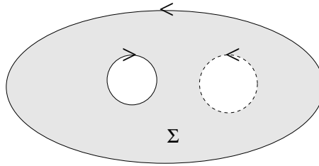
Fig. 4.15 A morphism \Sigma : C_1 \rightarrow C_2 .
